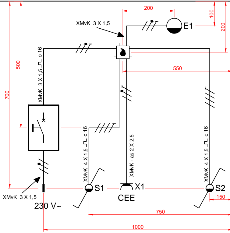
Installatieschema
