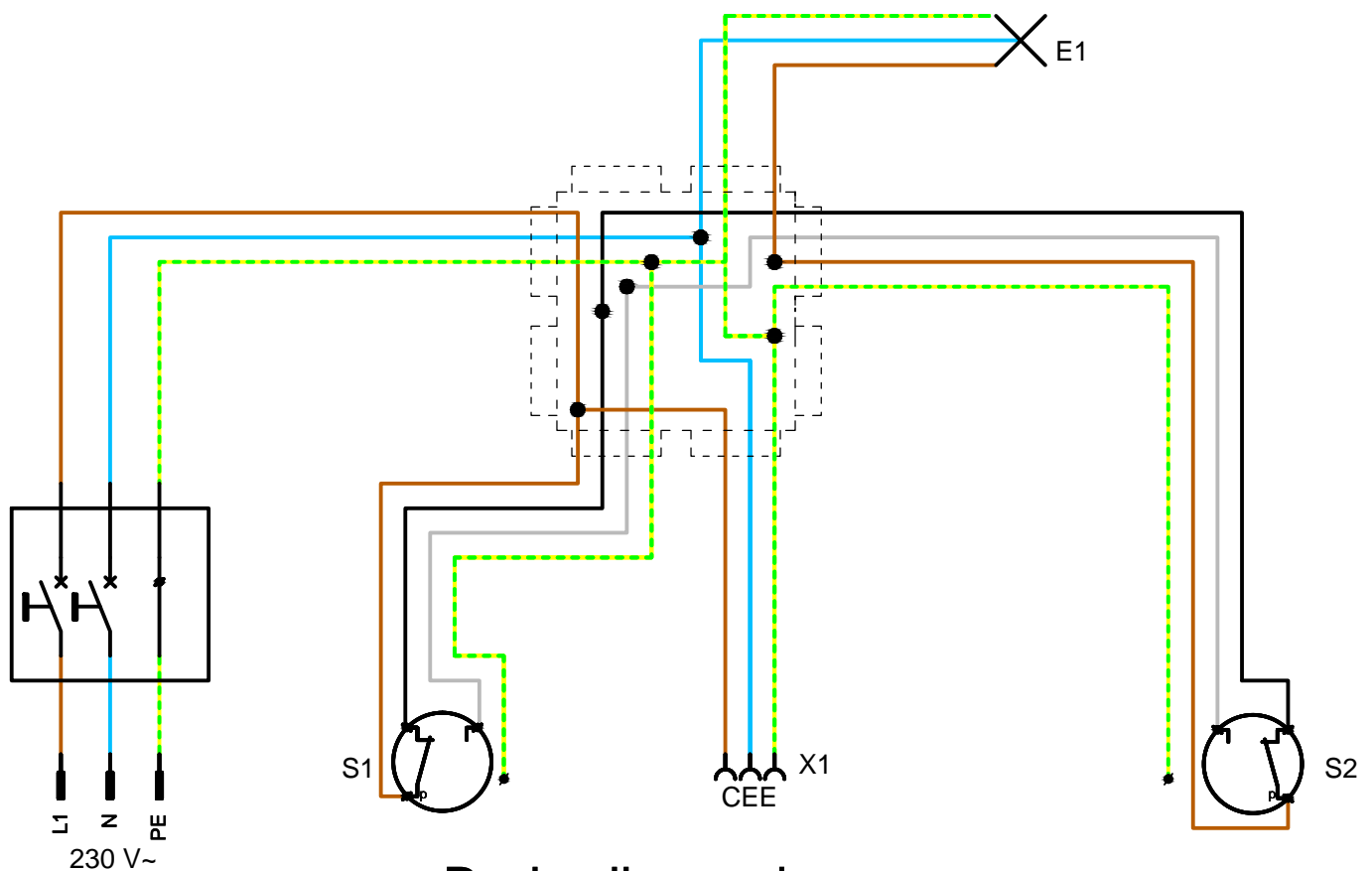
Bedradingschema
