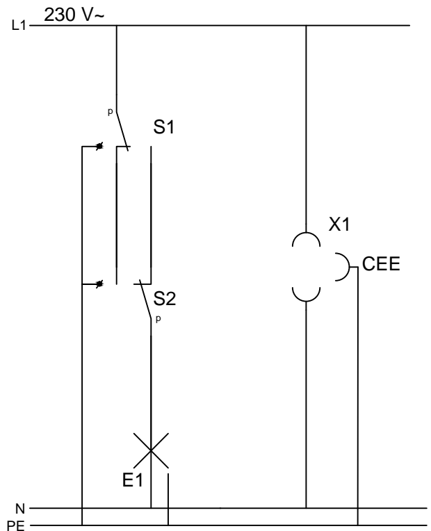
Stroomkringschema
